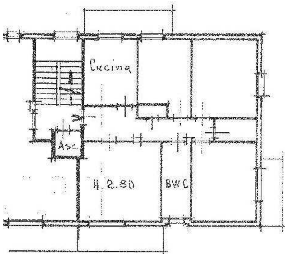
Planimetria alloggio oggetto di intervento, piano terzo (disegno fuori scala)
