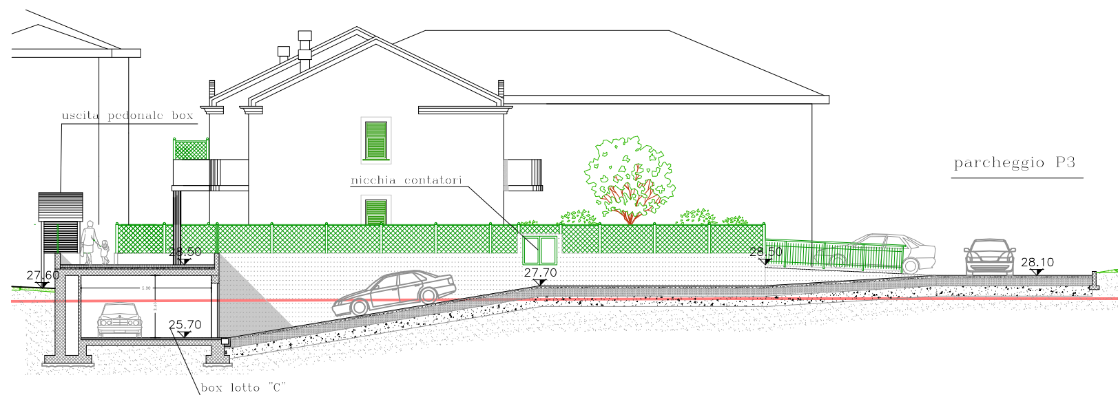
SEZIONE generale B-B (prosp. OVEST)
