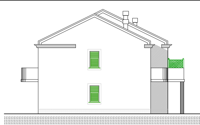
PROSPETTO EST
