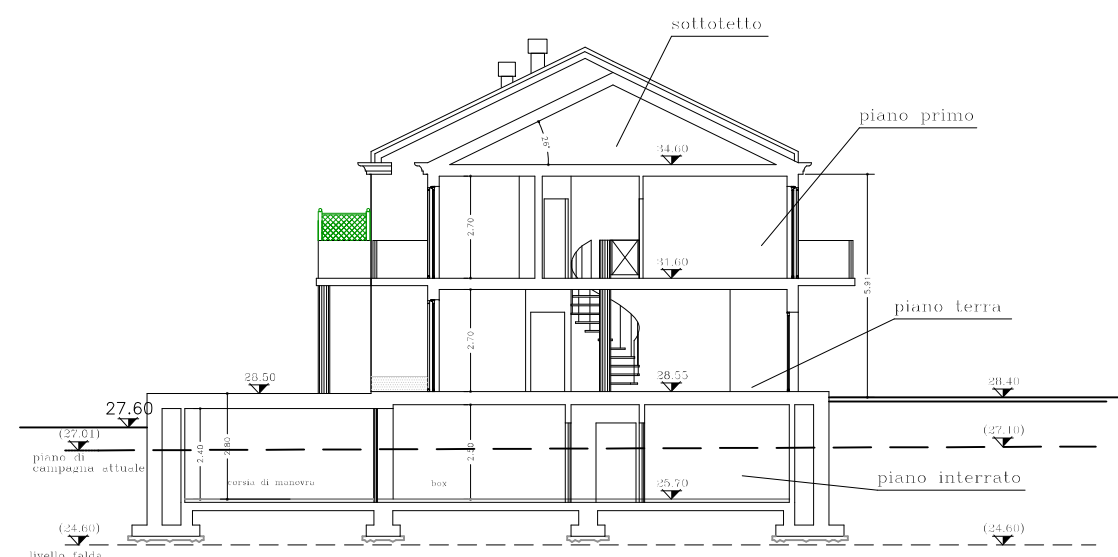
SEZIONE A-A
