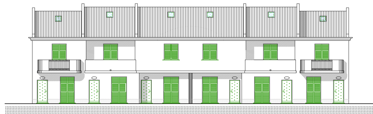
PROSPETTO SUD
