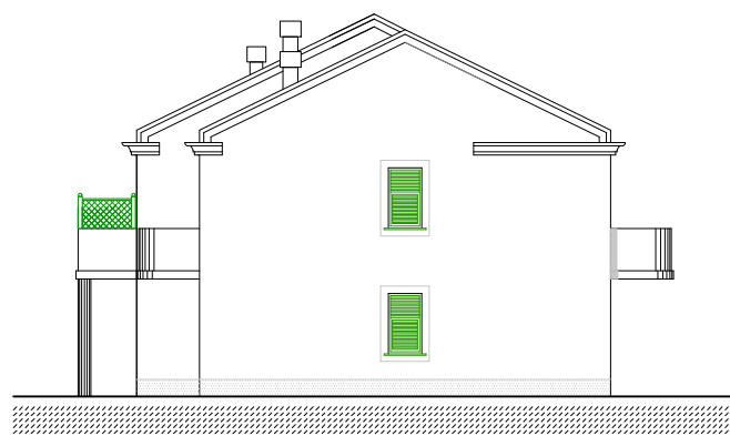
PROSPETTO OVEST
